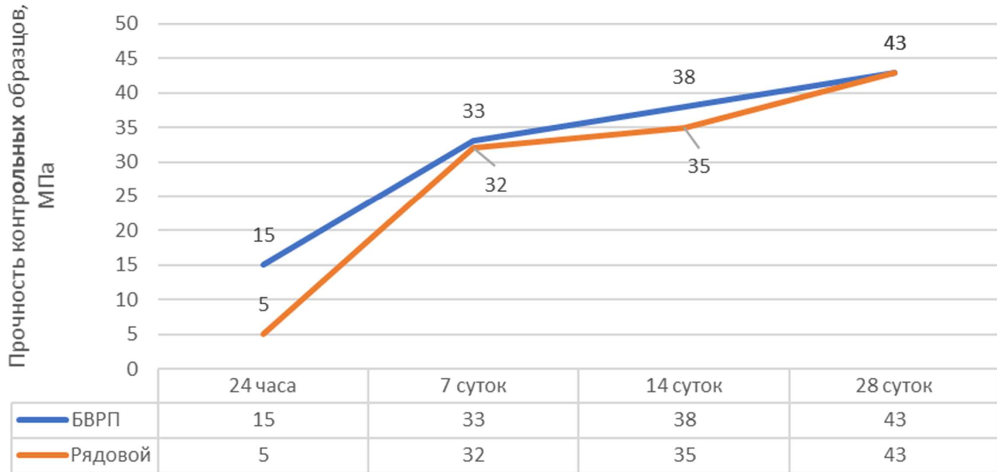
Сравнение прочности бетонов класса по прочности на сжатие В25 в разных возрастах
